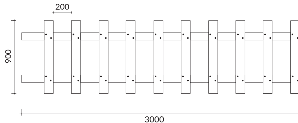
VISTA FRENTE
