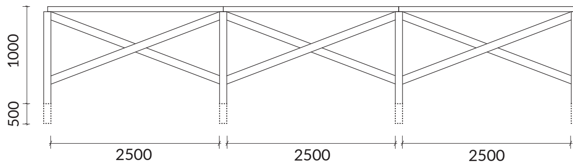
VISTA FRENTE
