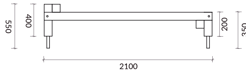
VISTA LATERAL
