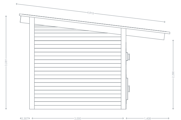
ALÇADO LATERAL
