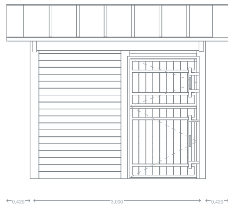
ALÇADO FRONTAL
