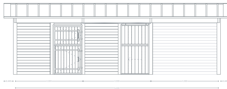
ALÇADO FRONTAL
