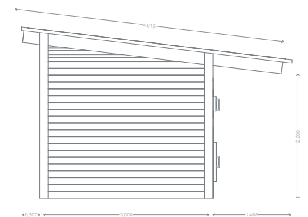
ALÇADO LATERAL
