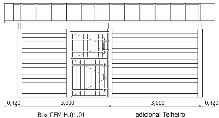
ALÇADO FRONTAL
