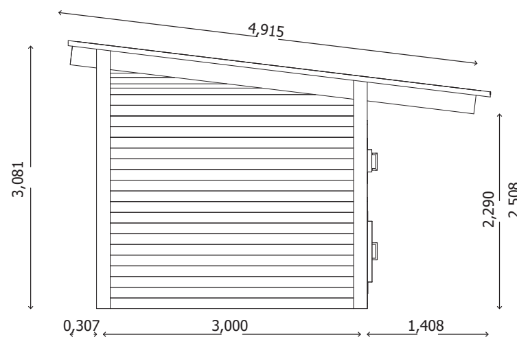
ALÇADO LATERAL
