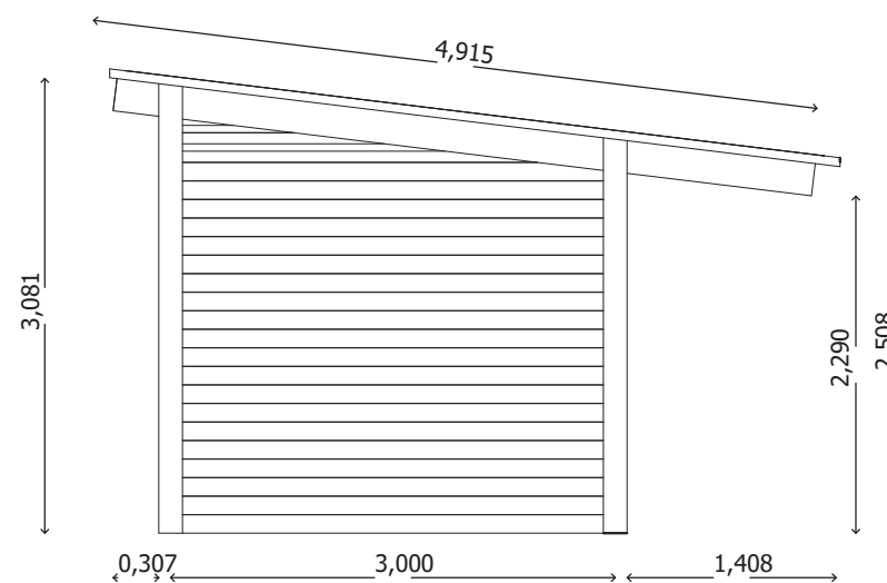
ALÇADO LATERAL
