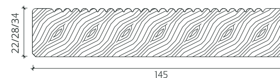
DESENHO TÉCNICO
